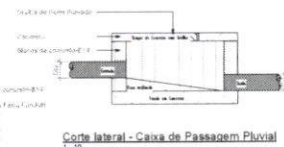
11 Corte lateral - Caixa de Passagem Pluvial
