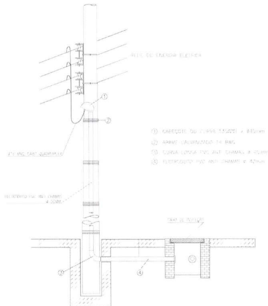
RAMAL DE LIGAÇÃO SEM ESCALA
